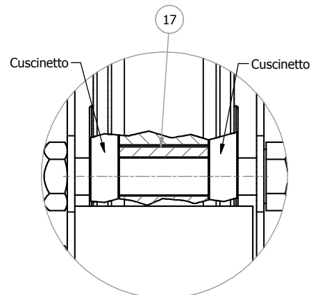
Dettaglio C Scala 1 : 1
